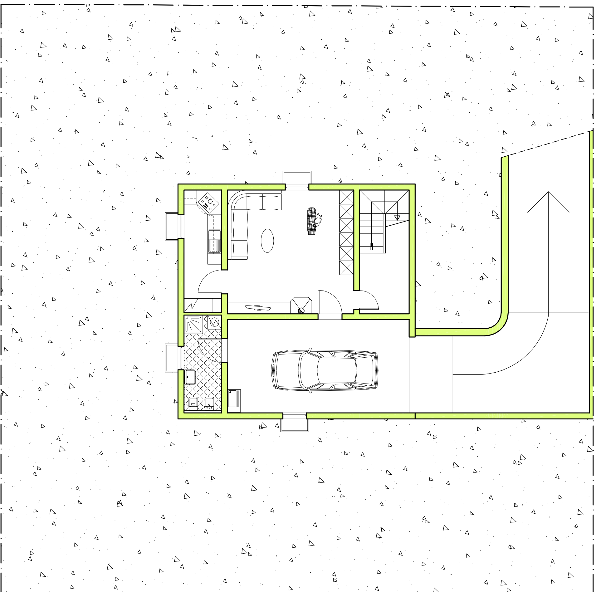
LOTTO 6 PIANTA PIANO SEMINTERRATO con ipotesi di arredo
