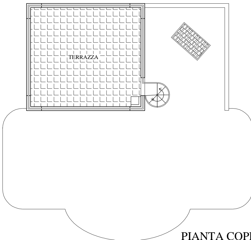
PIANTA COPERTURA
